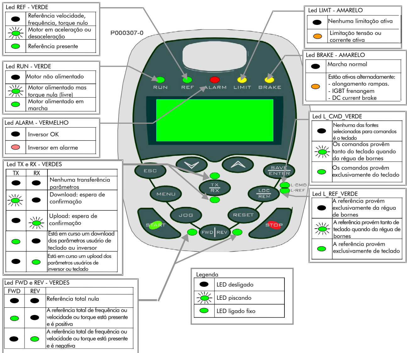
Figura 64: Módulo display
