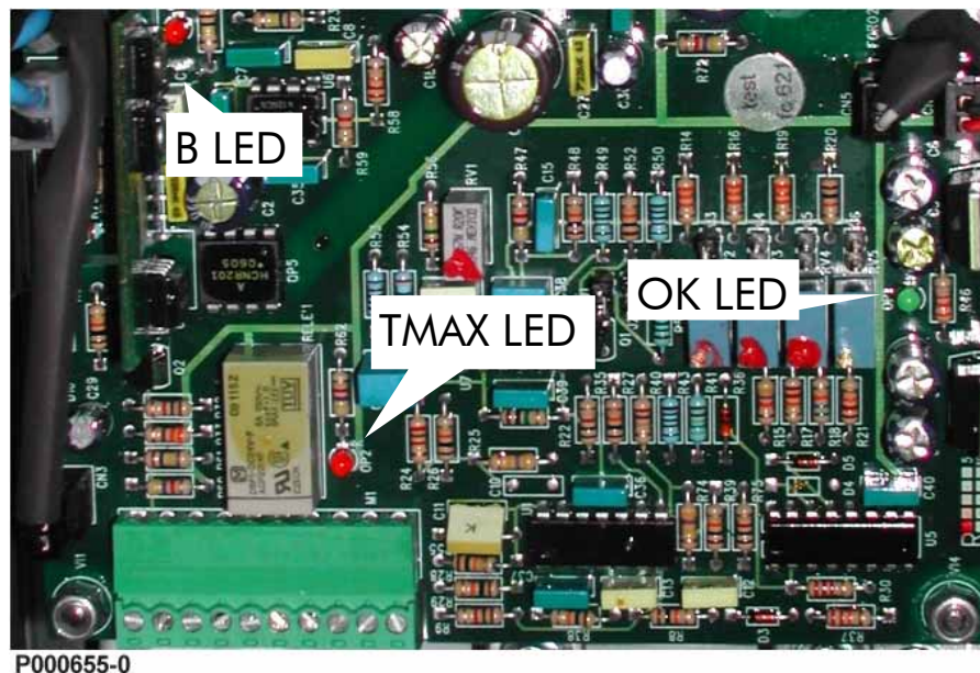
Figura 73: Posição dos LEDs de sinalização
