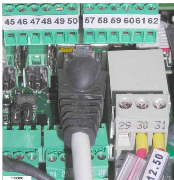
Figura 156: Cablagem cabo Ethernet
