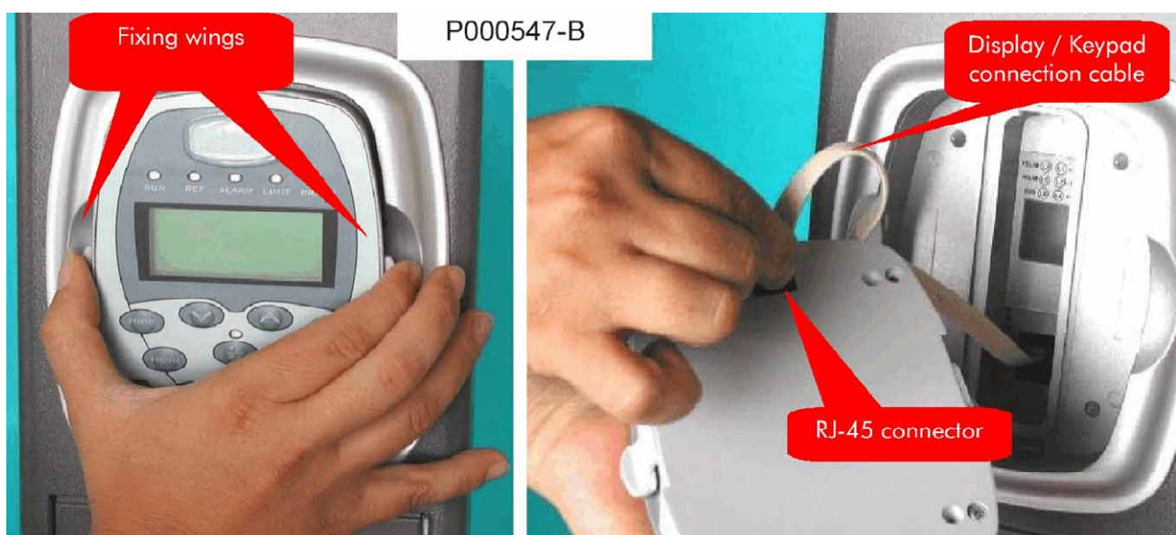
Figura 65: Remoção módulo teclado
