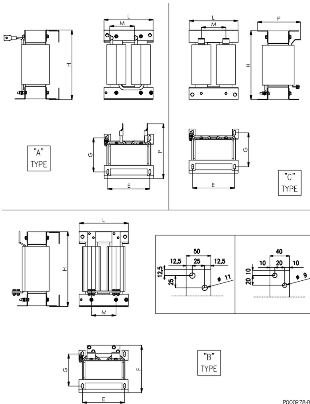
Figura 100: Características mecânicas Indutância DC
