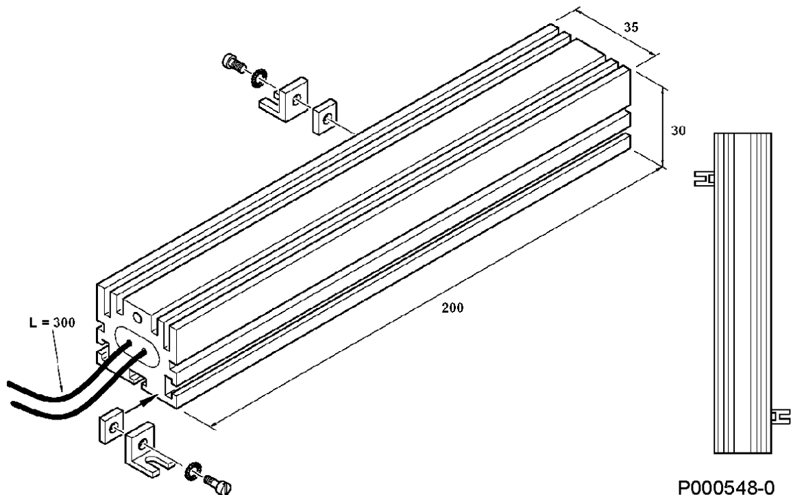
Figura 88: Dimensões de volume resistência 56-100Ω/350W
