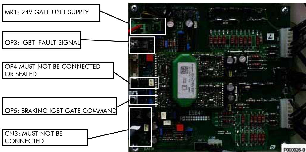
Figura 85: ES841 Placa gate unit módulo de frenagem
