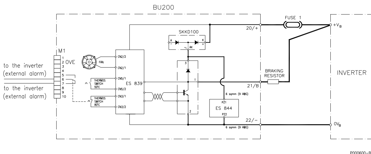
Figura 76: Ligação BU200 ao inversor em configuração individual
