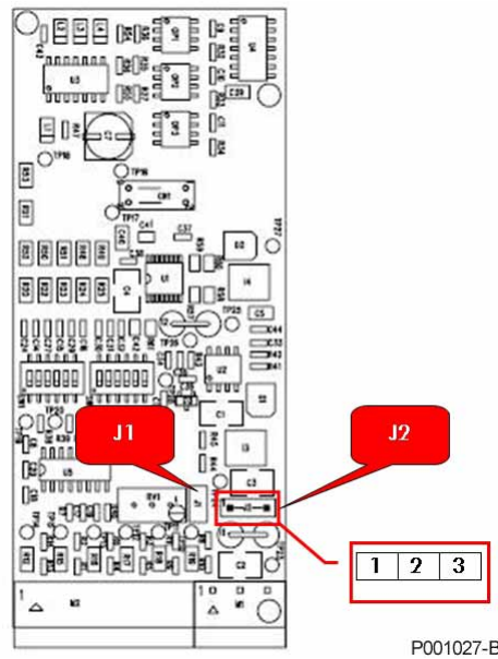
Figura 118: Posição dos jumpers de seleção da tensão de alimentação encoder
