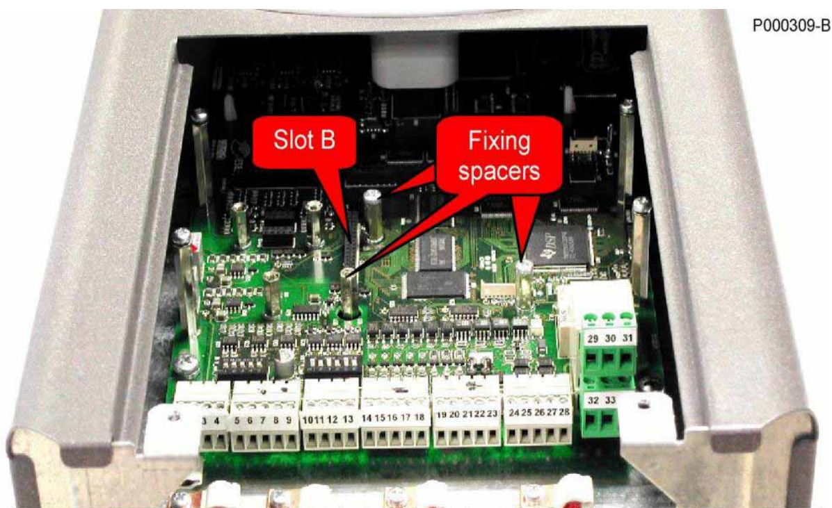
Figura 142: Posição do slot para inserção placa ES919
