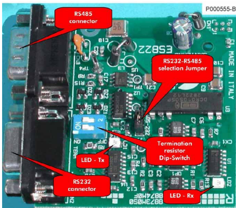
Figura 119: Placa ES822
