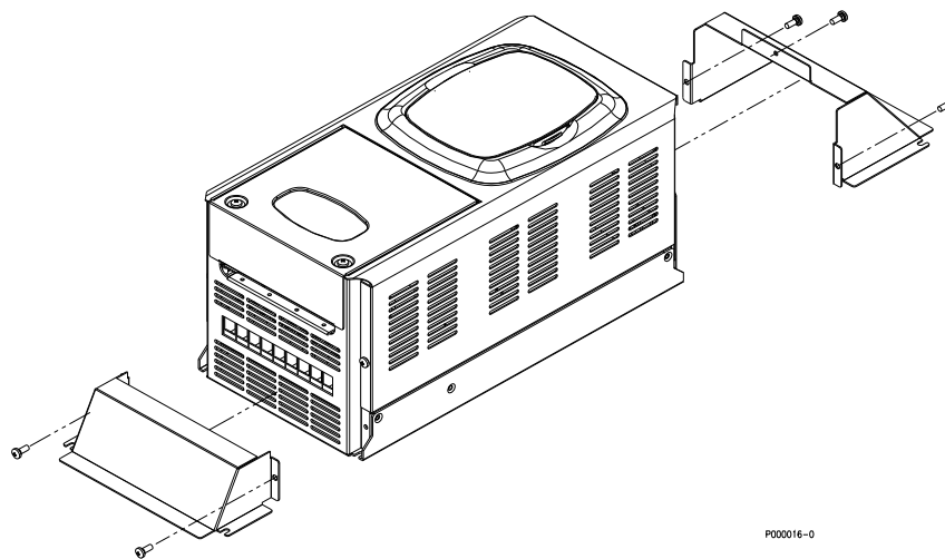
Figura 5: Aplicação acessórios para a montagem passante SINUS PENTA S05
