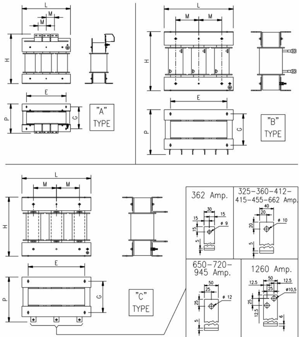
Figura 99: Características mecânicas indutância trifásica
