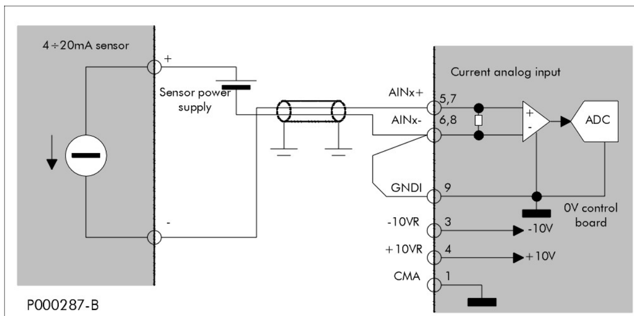
Figura 57: Ligação sensor 4÷20mA
