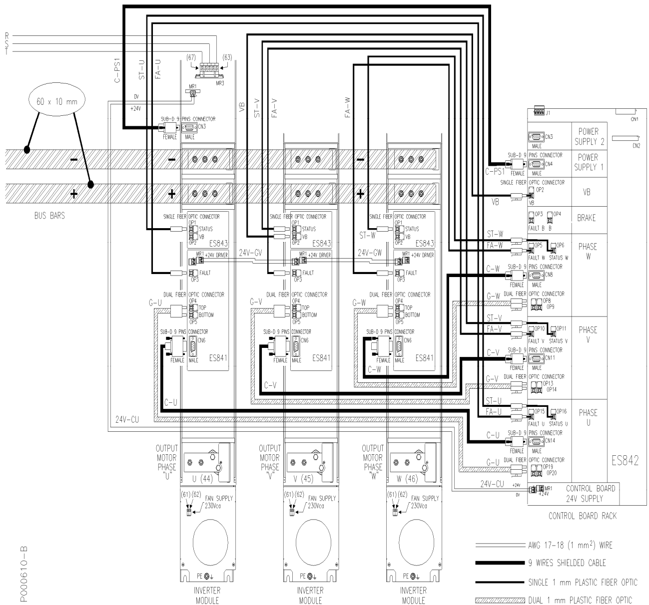
Figura 38: Ligações internas inversor S64
