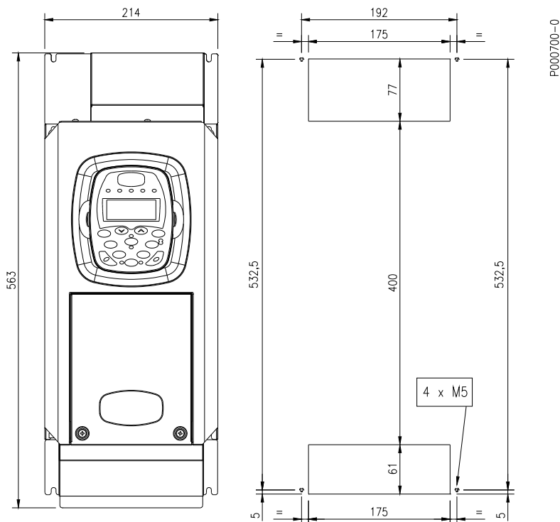
Figura 8: Dimensão de furação do painel para montagem passante SINUS PENTA S12
