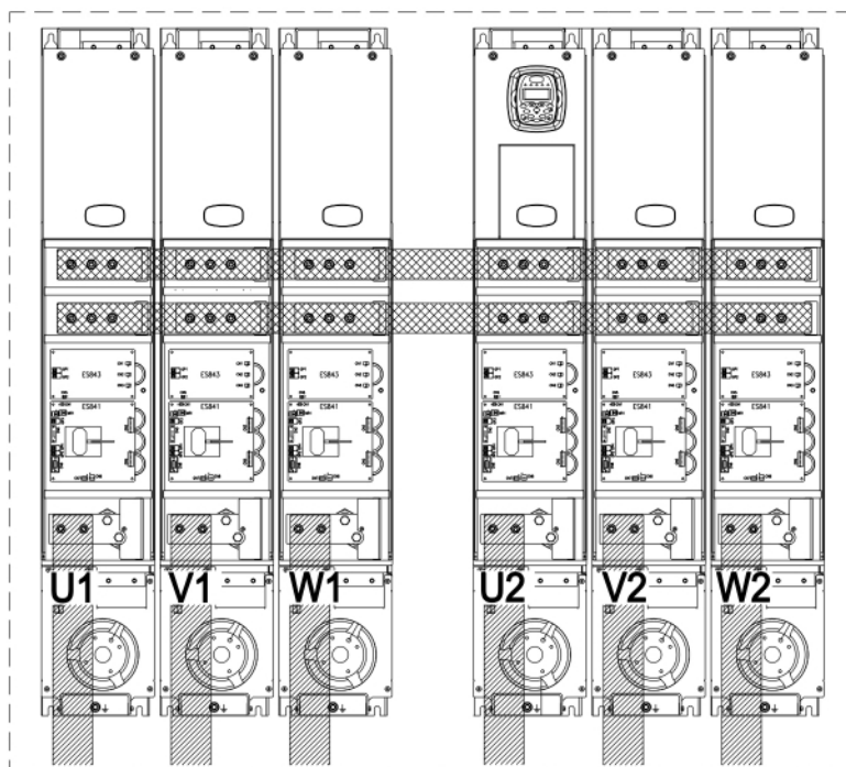
Figura 42: Barras de ligação S74
