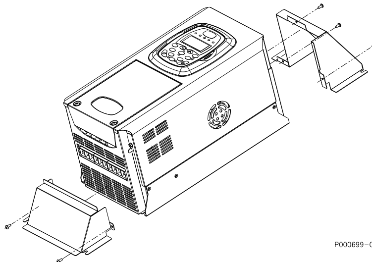
Figura 7: Aplicação acessórios para a montagem passante SINUS PENTA S12
