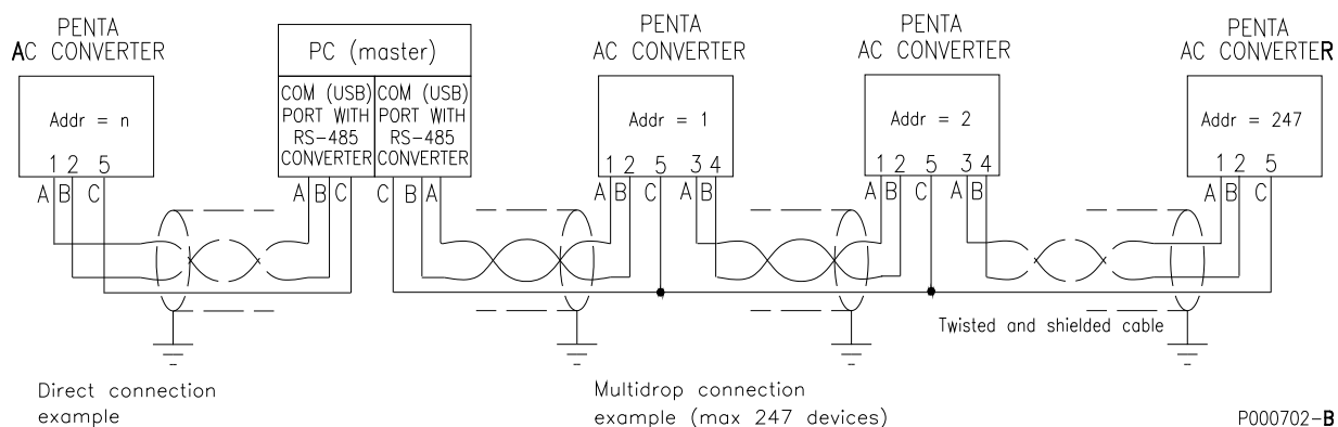
Figura 67: Exemplo de conexão direta e multidrop
