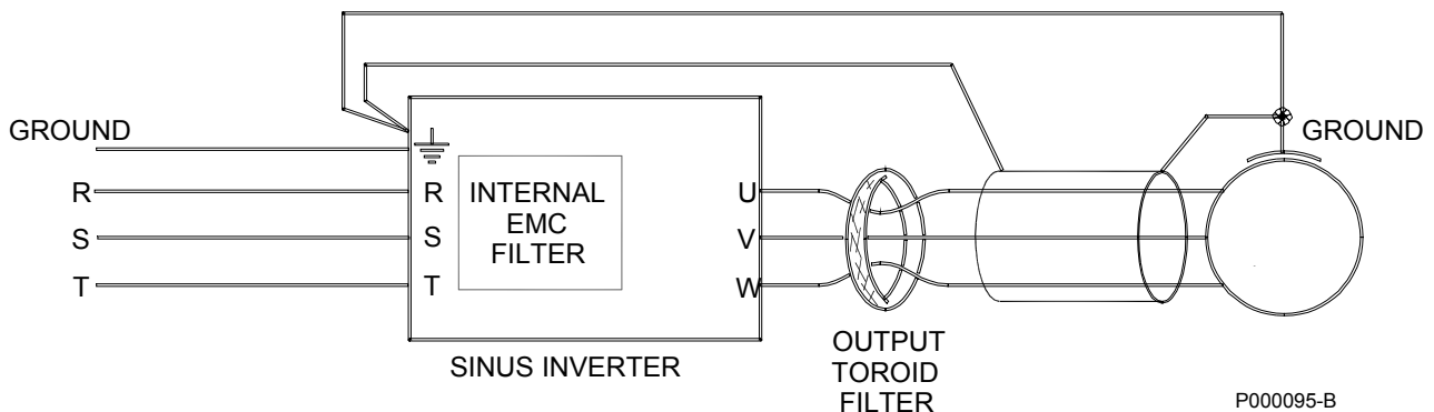
Figura 177: Ligação filtro toroidal para SINUS PENTA
