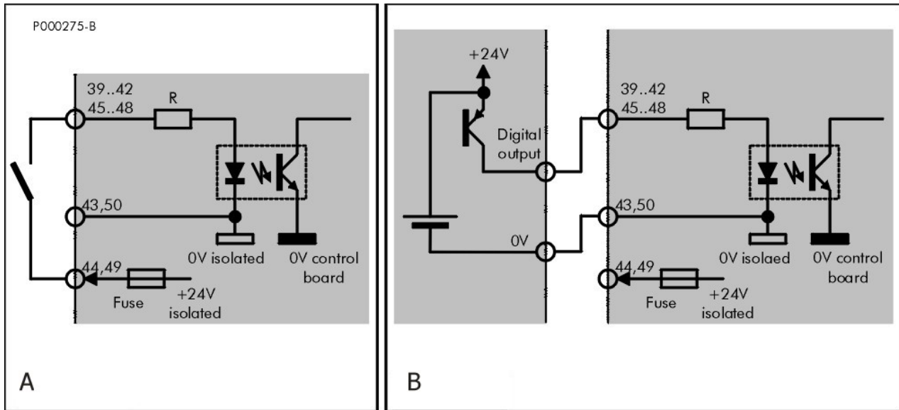
Figura 164: Ligação de entradas de tipo PNP
