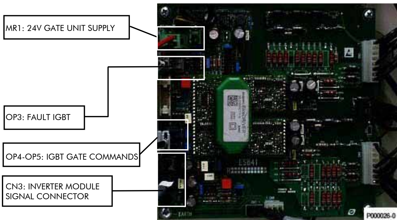
Figura 33: ES841 Placa gate unit modulo inversor
