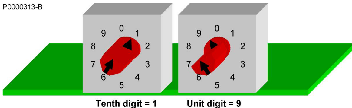
Figura 128: Exemplo de posicionamento dos rotary-switchs para ajustar o endereço Profibus 19.
