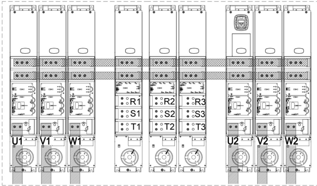
Figura 20: Exemplo di instalação de um SINUS PENTA S75/S80 (S75 tem dois módulos alimentador)
