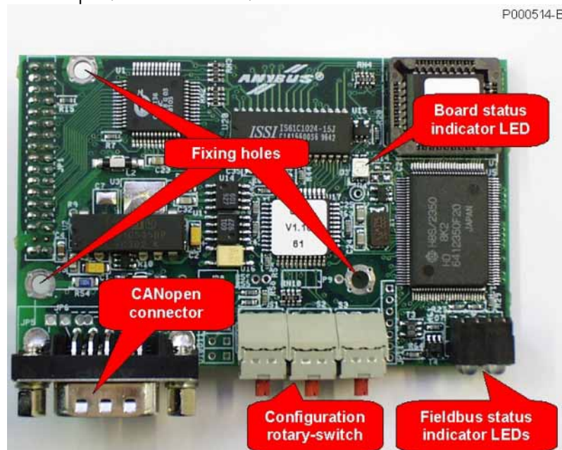
Figura 131: Placa comunicação fieldbus CANOpen
