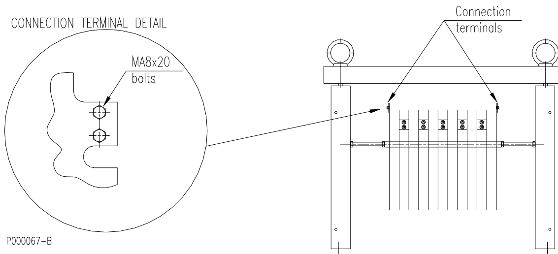
Figura 93: Localizações conexões elétricas resistências em caixa
