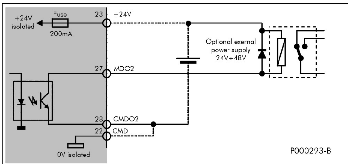
Figura 63: Ligação saída NPN para comando a relê
