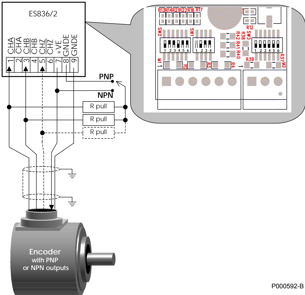
Figura 111: Encoder tipo PNP ou NPN com saídas single-ended e resistências de carga cabladas externamente
