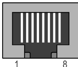
Figura 68: Disposição pin do conector teclado / linha serial 1
