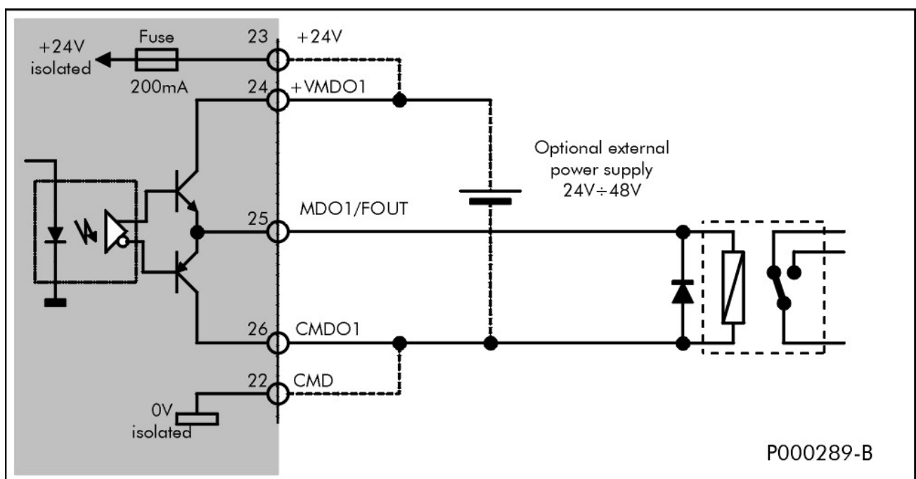
Figura 59: Ligação saída PNP para comando relè
