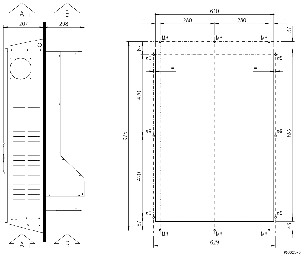
Figura 13: Montagem passante e relativas dimensões de furação para SINUS PENTA S50
