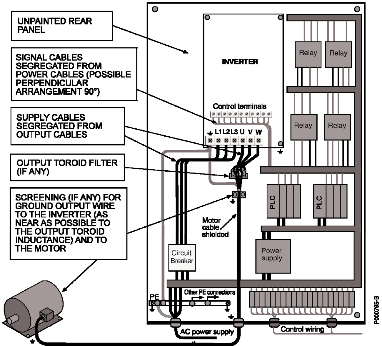
Figura 176: Exemplo di correto cablagem de um inversor em quadro
