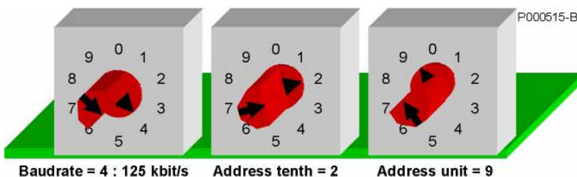
Figura 132: Exemplo de posicionamento dos rotary-switches para 125kbit/s e Device Address 29.
