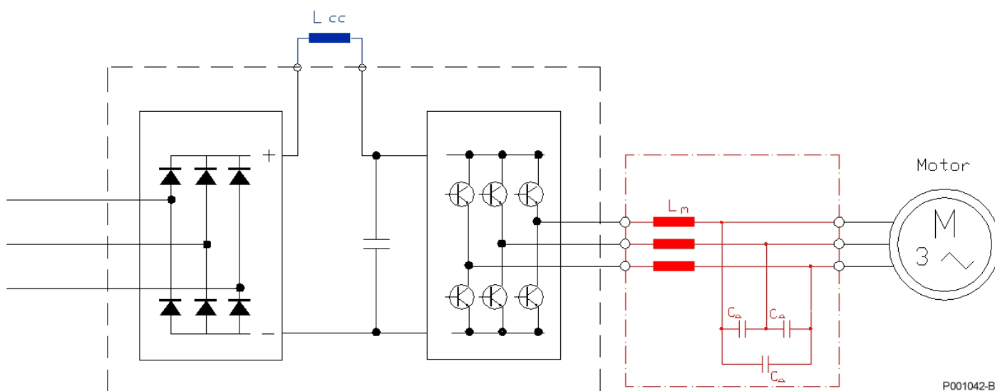
Figura 104: Filtro sinusoidal
