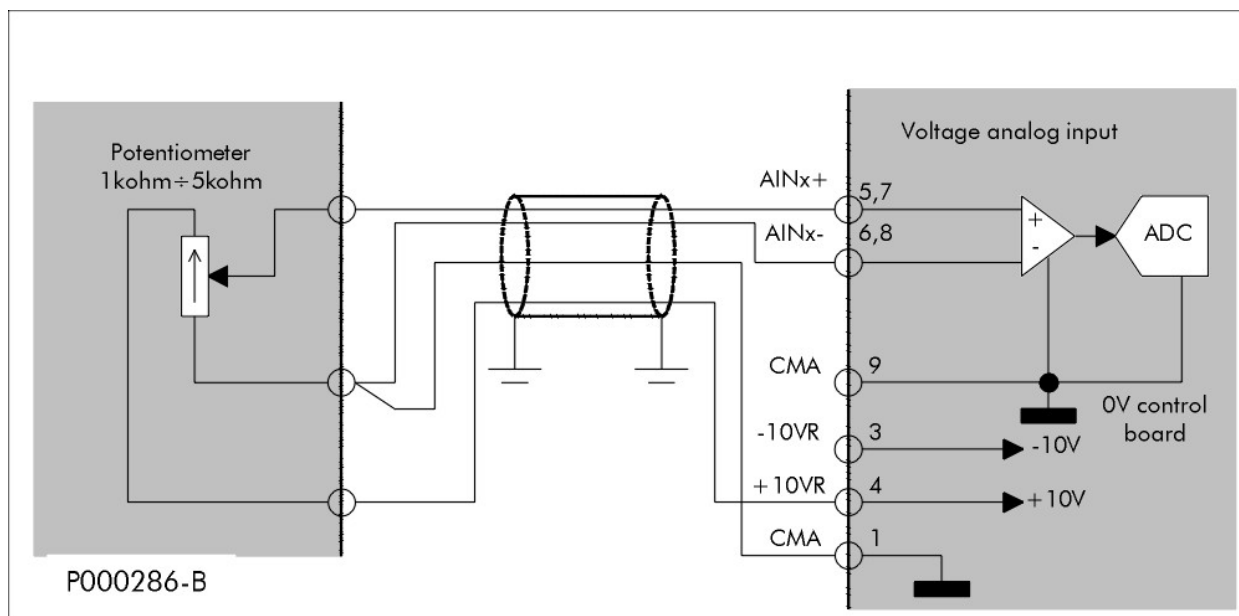
Figura 56: Ligação potenciômetro remoto unipolar 0+REFmax
