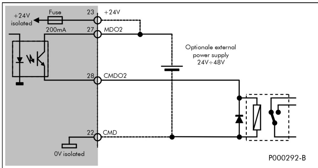
Figura 62: Ligação saída PNP para comando relê
